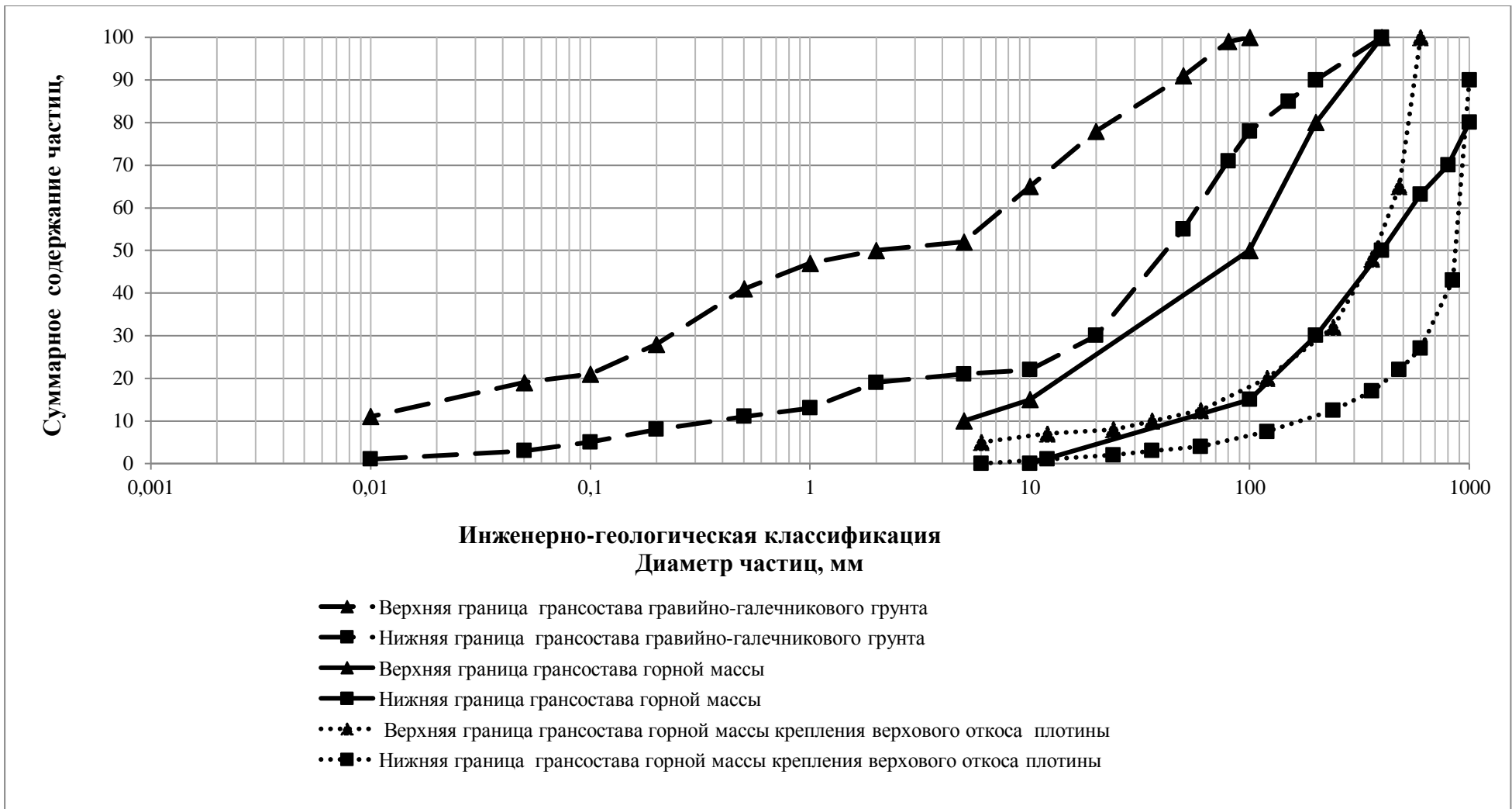
Рисунок 3.8.2.1 - Гранулометрические составы грунтов, пригодных для укладки в правобережную каменно-земляную плотину во II понижении
